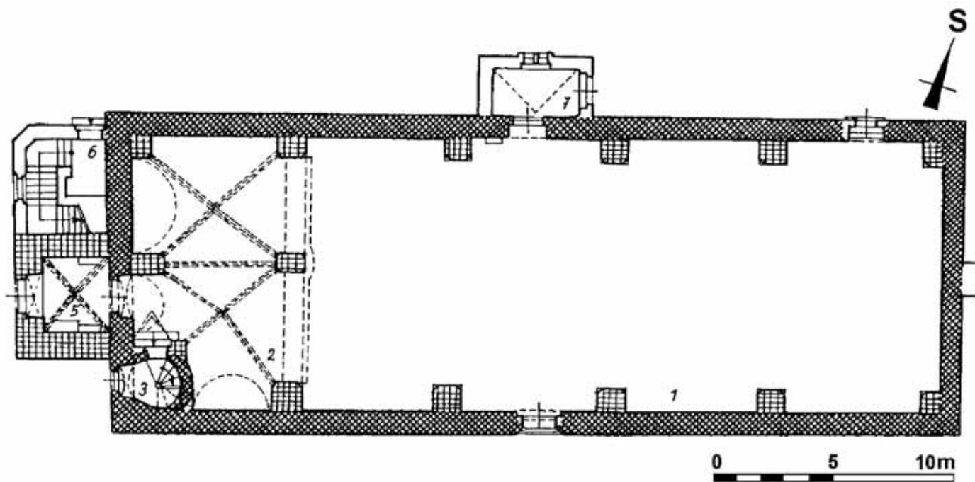
Obr. 2 Stavebně historický průzkum kostela sv. Markéty ve Strakonících podle F. Kašičky z roku 1996. Jádru objektu tvoří obdélná hala středověkého johanitského špitálu pocházející pravděpodobně z období 1442–1462.
